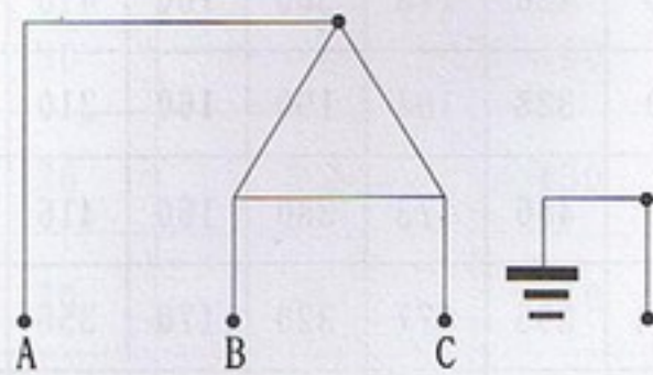
角型接线图
