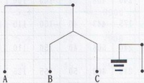
星型接线图
